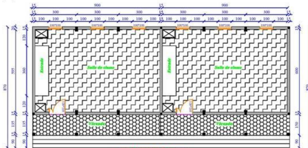
Plan de construction d'un bloc de 2 classes
