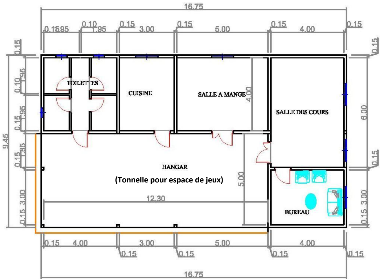
Plan du jardin d'enfants : Coût 22300 €
